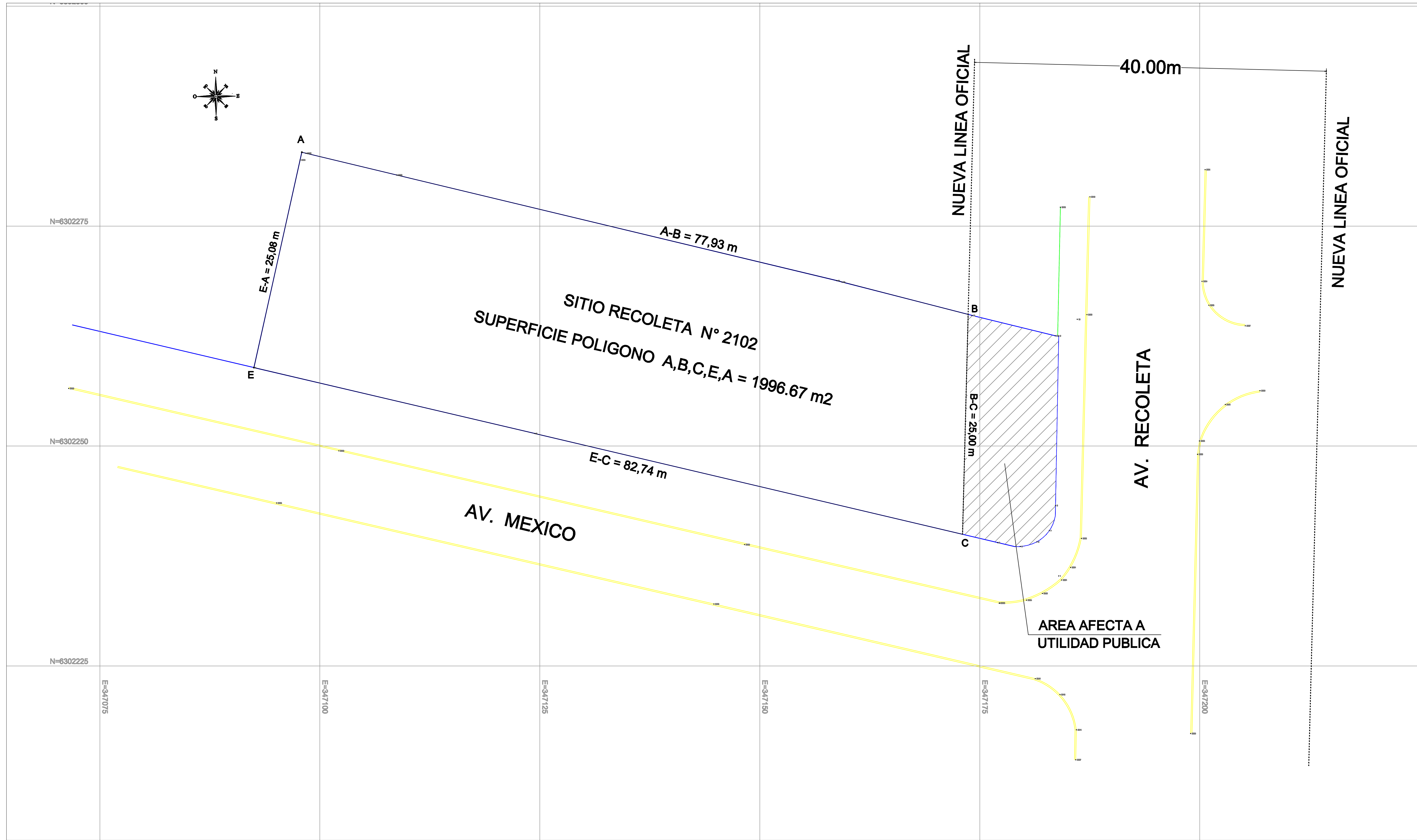
PLANO PLANTA ESC. 1:200
